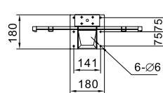
BBS35VT-1000
